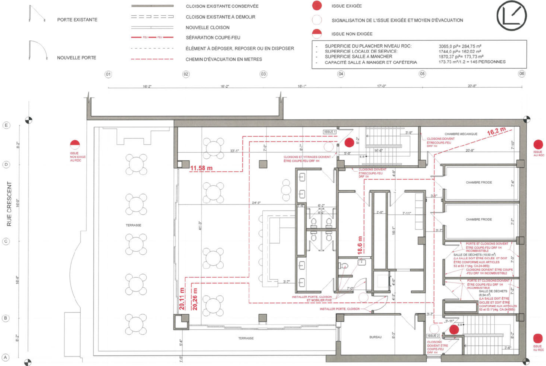
1 PLAN PROPOSÉ 3ÈME ÉTAGE (SUITE: 1476-C) A-06 ECHELLE: 1/8" = 1'-0"
